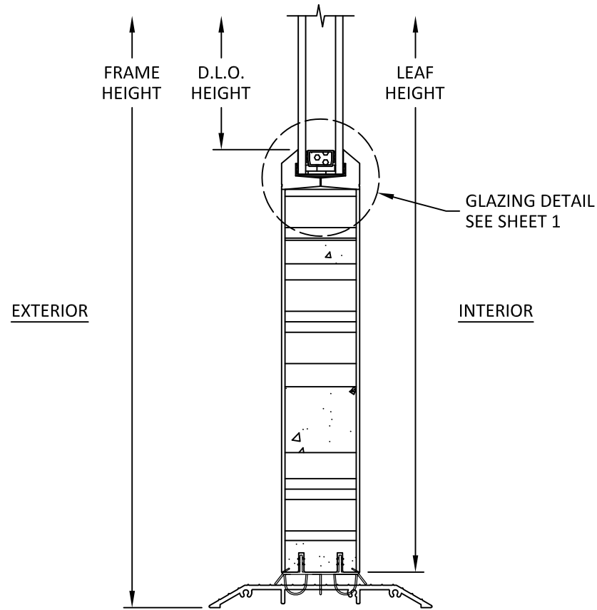
C 3 VERTICAL SECTION DOOR ADA SILL *
